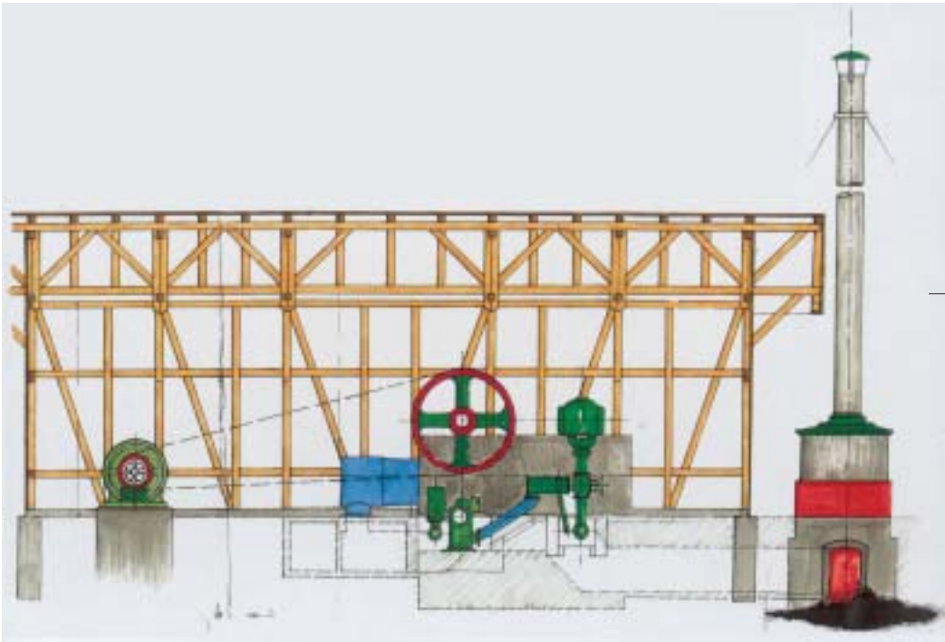
Plan des E-Werks am Heufurtweg
